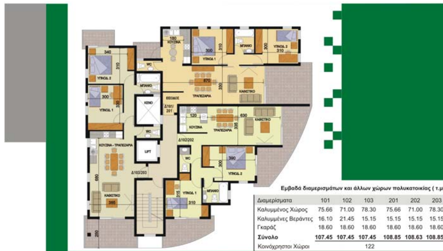
Τυπική Κάτοψη ορόφων πολυκατοικίας
